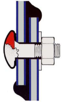
Verschraubung / Eindingung der Segmentplatten
